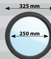
Attraktive runde Fenster
